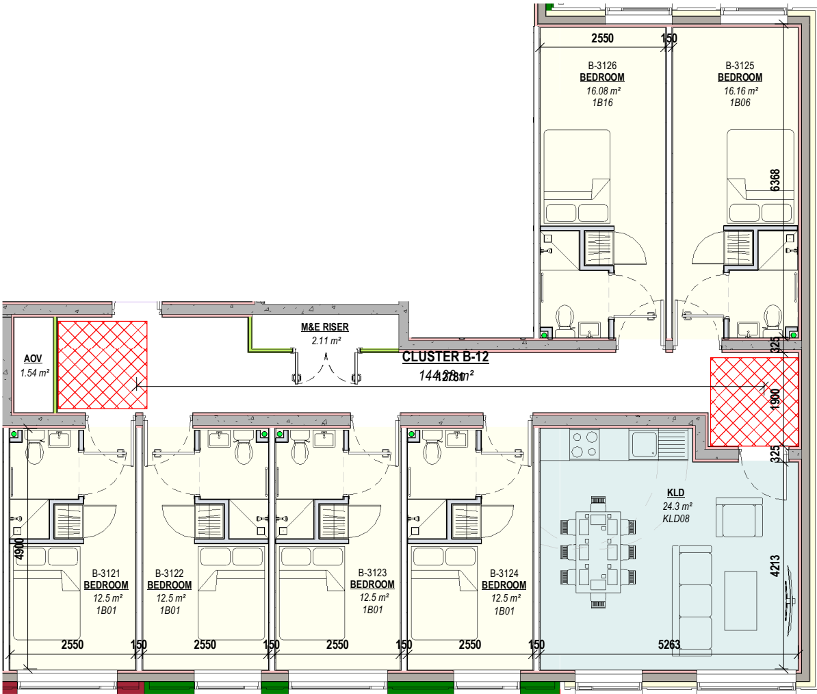
2 CLUSTER B-12 Scale: 1 : 100
