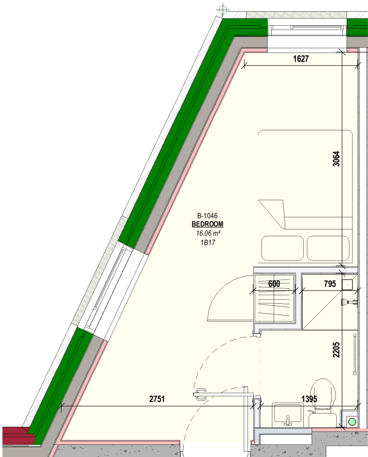
2 1B17 Scale: 1 : 50
