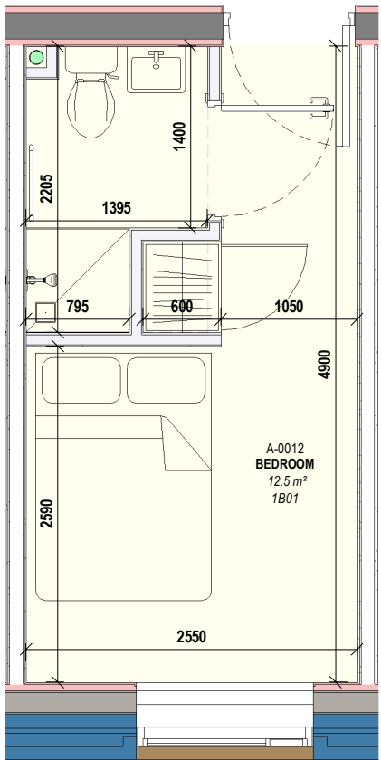
1 1 Bed Type 1B01 Scale: 1 : 50
