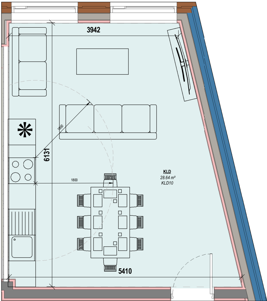
2 KLD10 Scale: 1 : 50
