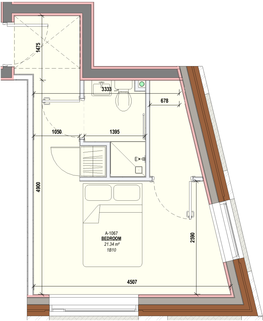
2 1B10 Scale: 1 : 50
