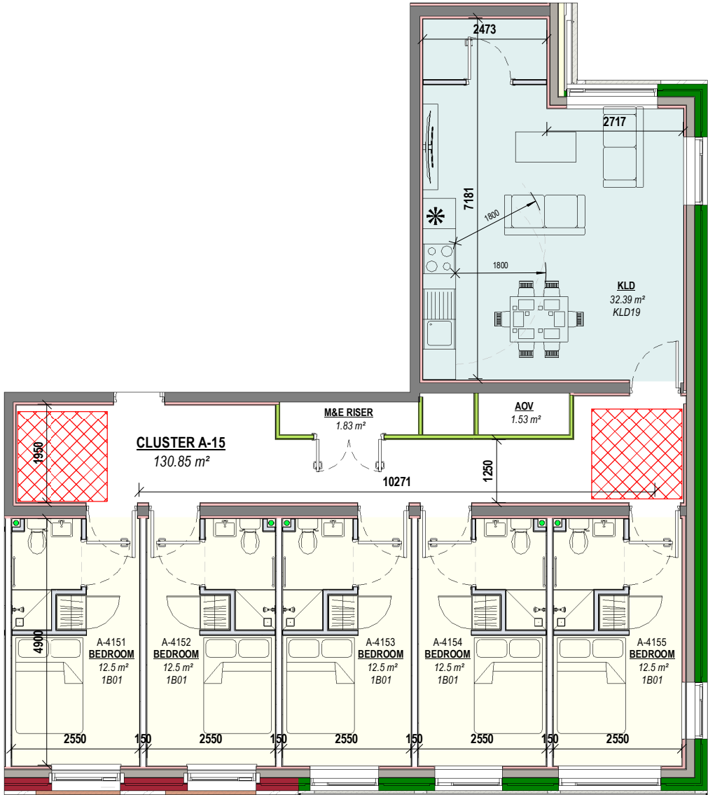
1 CLUSTER A-15 Scale: 1 : 100
