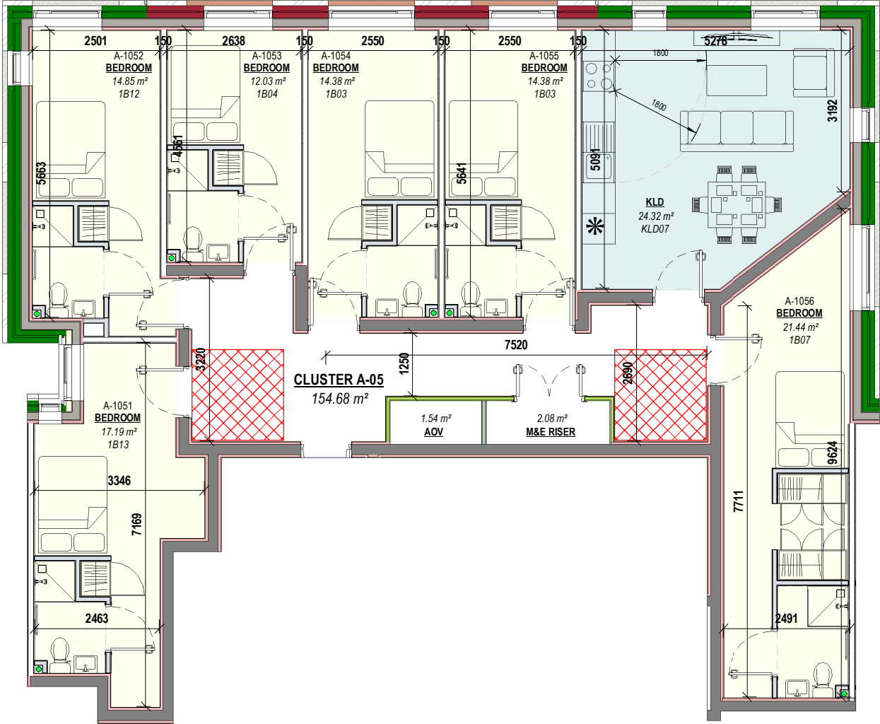
1 CLUSTER A-05 Scale: 1 : 100
