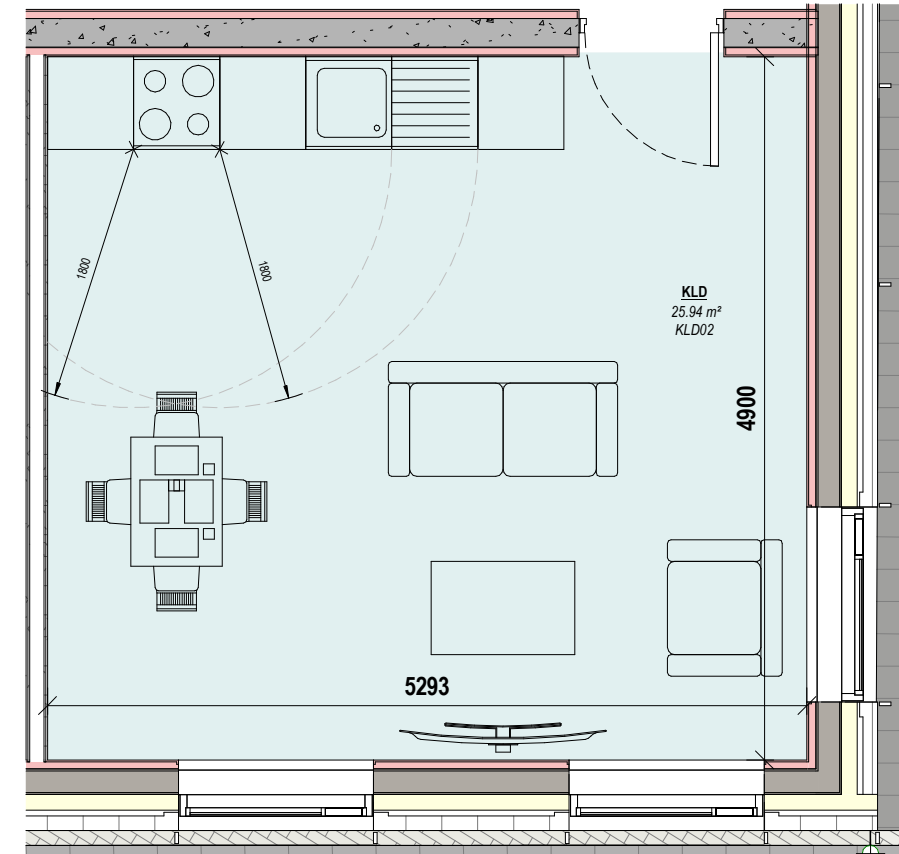
2 KLD02 Scale: 1 : 50
