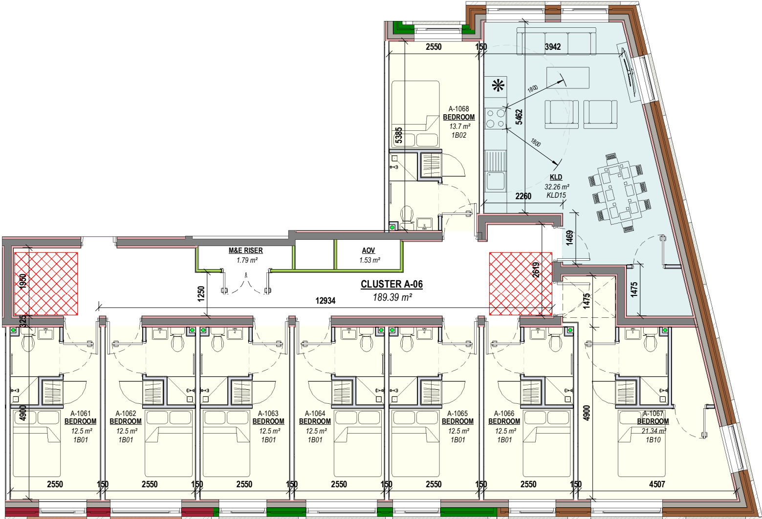
1 CLUSTER A-06 Scale: 1 : 100
