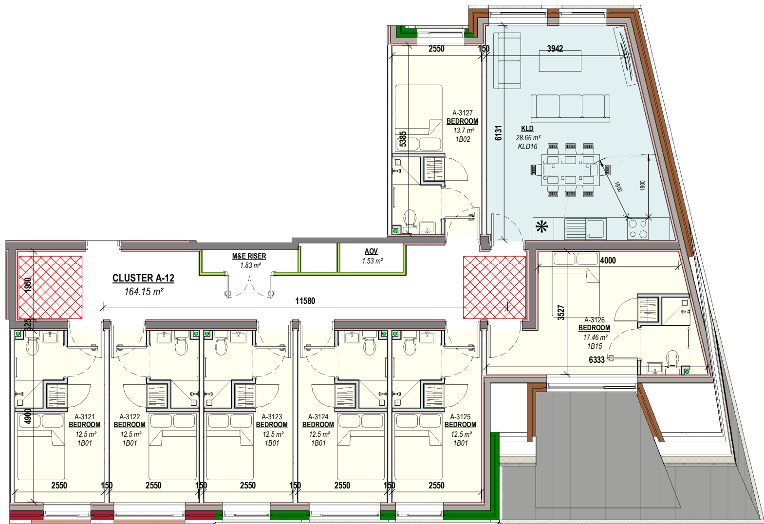
1 CLUSTER A-12 Scale: 1 : 100
