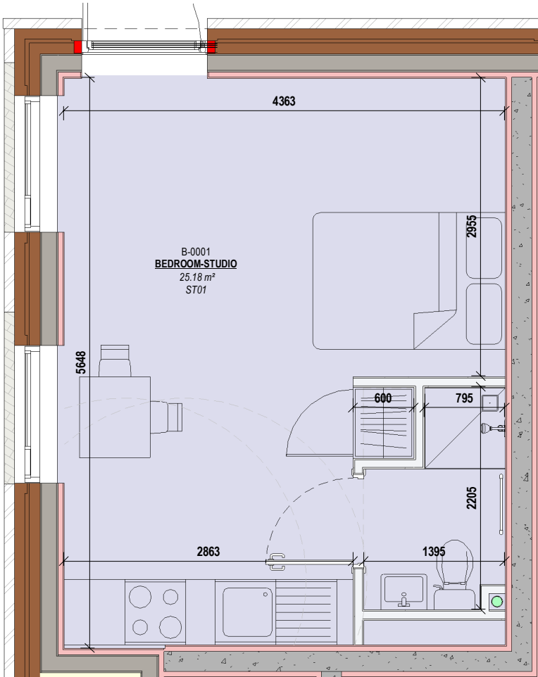
4 ST01 Scale: 1 : 50
