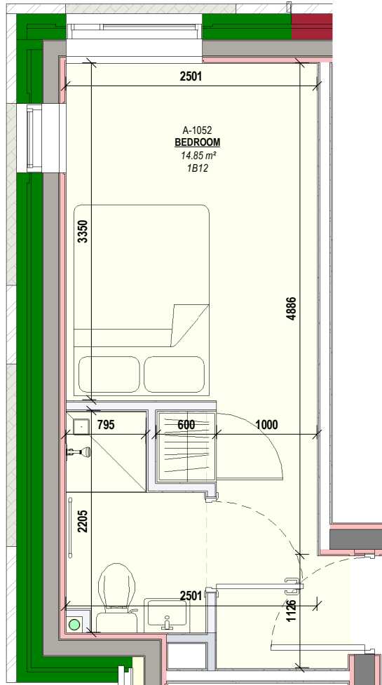
1 1B12 Scale: 1 : 50
