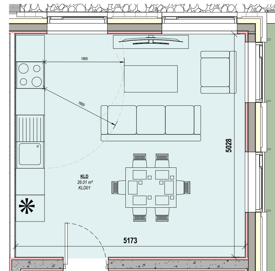
1 KLD01 Scale: 1 : 50
