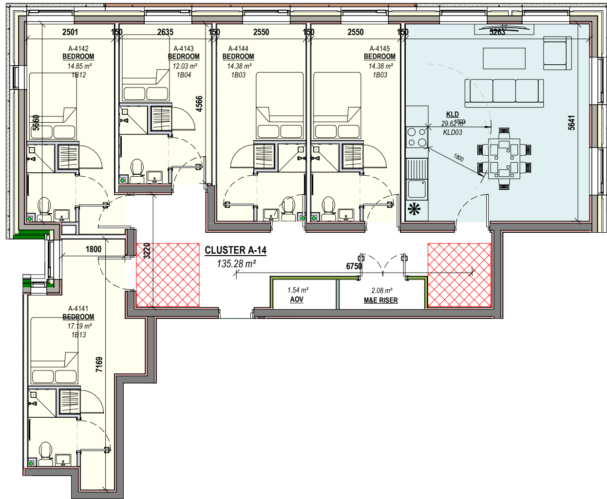
1 CLUSTER A-14 Scale: 1 : 100
