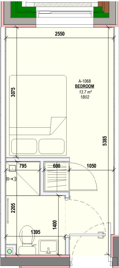
2 1 Bed Type 1B02 Scale: 1 : 50
