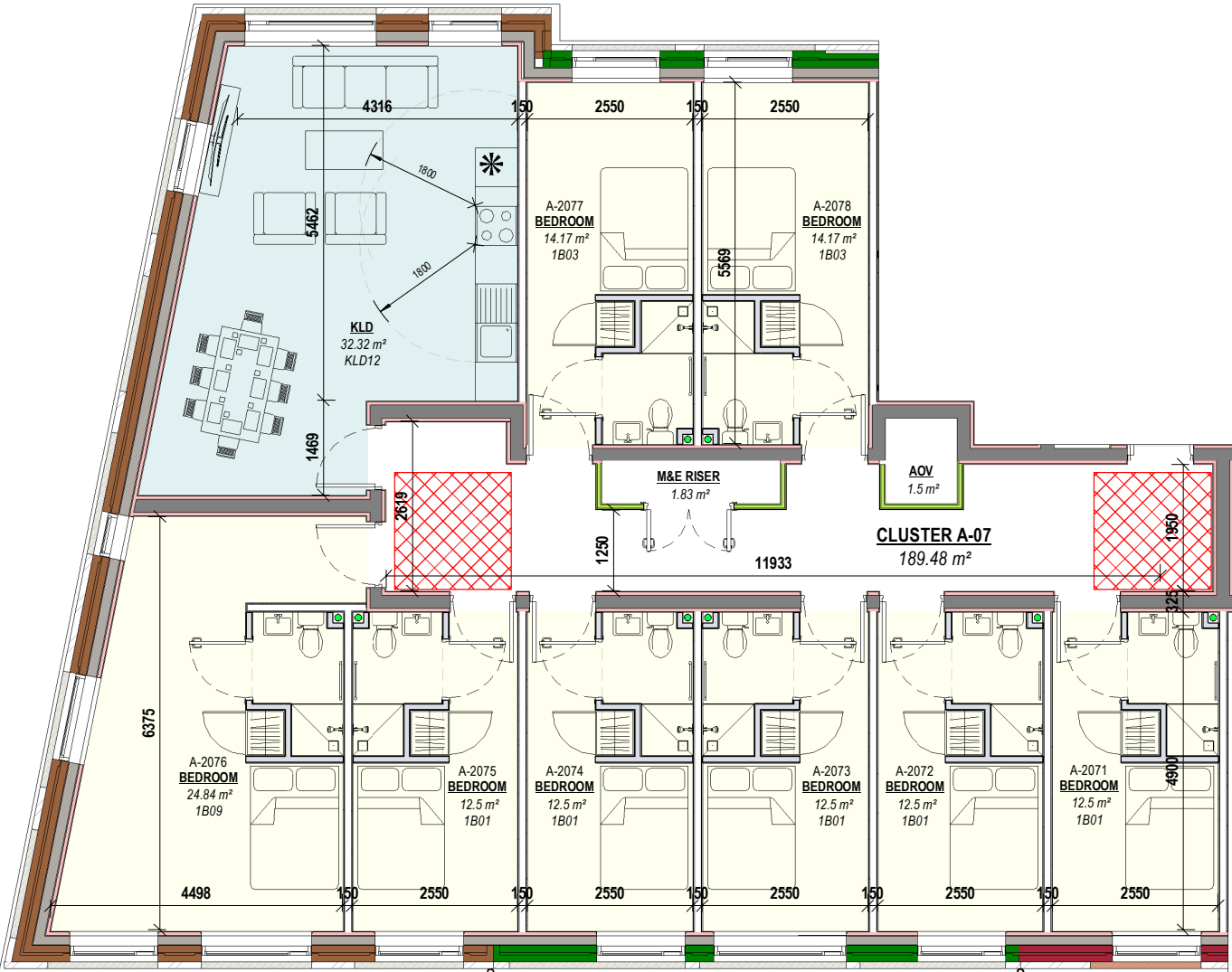
1 CLUSTER A-07 Scale: 1 : 100
