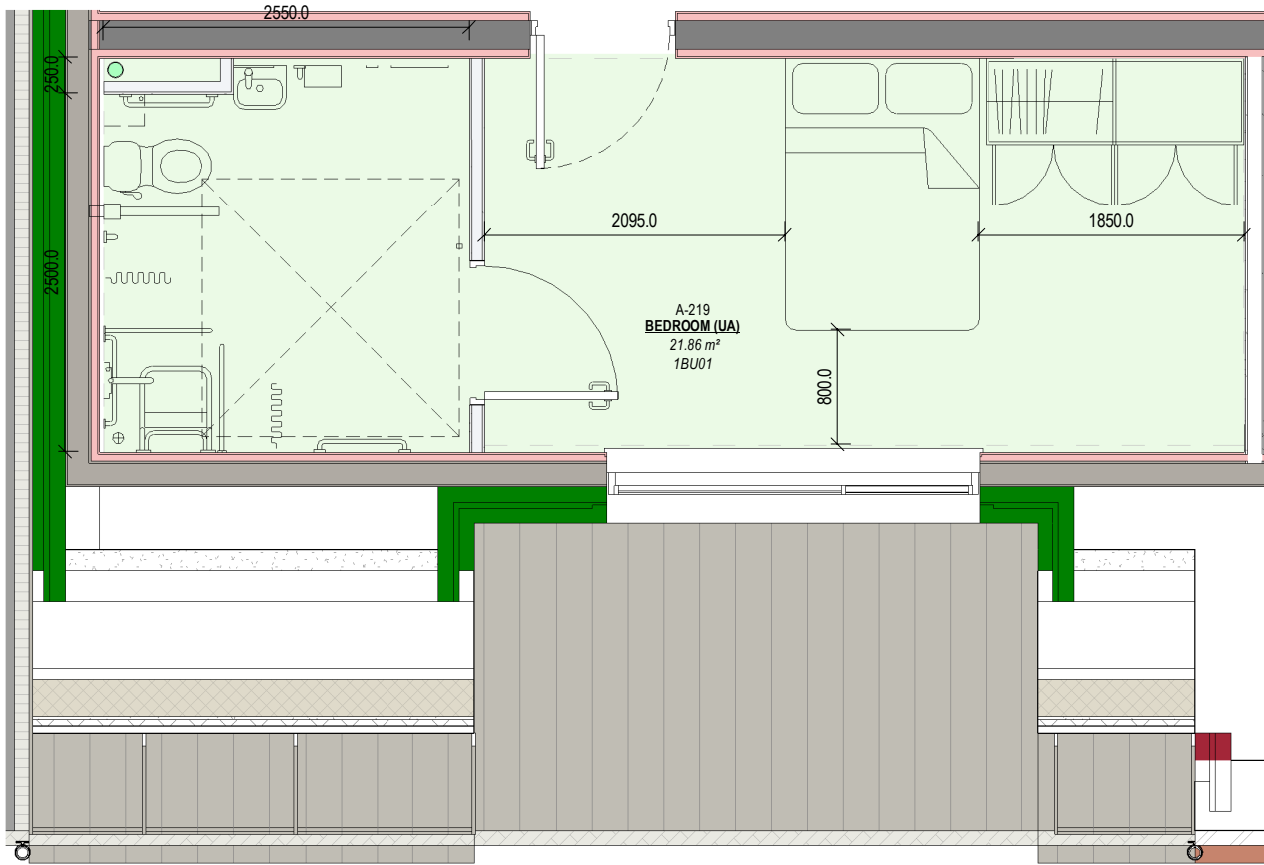
1 1BU01 Scale: 1 : 50
