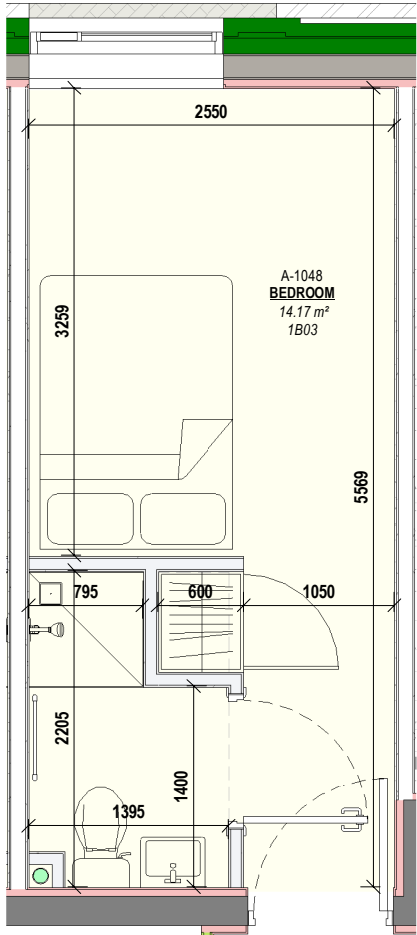
3 1 Bed Type 1B03 Scale: 1 : 50
