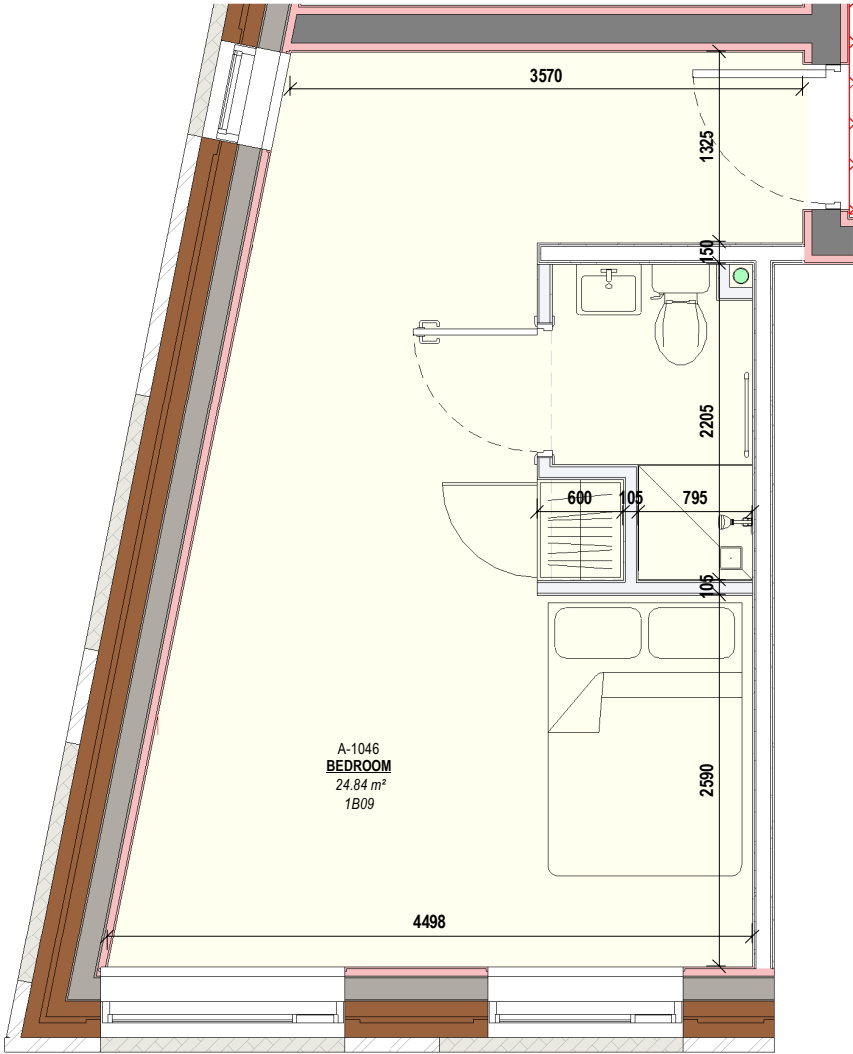
1 1B09 Scale: 1 : 50
