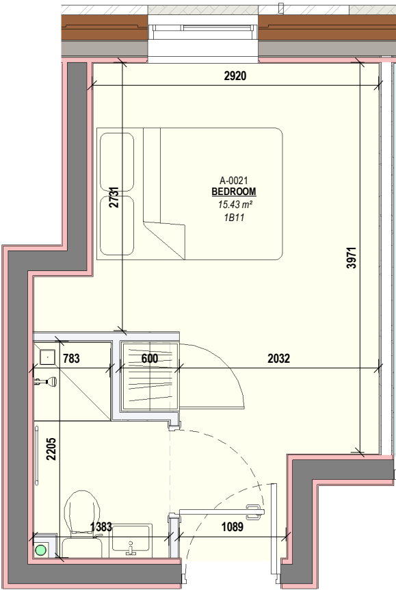
3 1B11 Scale: 1 : 50
