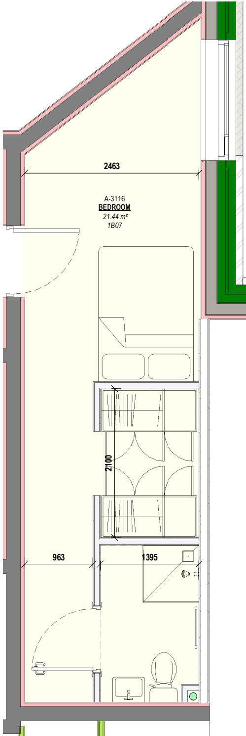
3 1B07 Scale: 1 : 50
