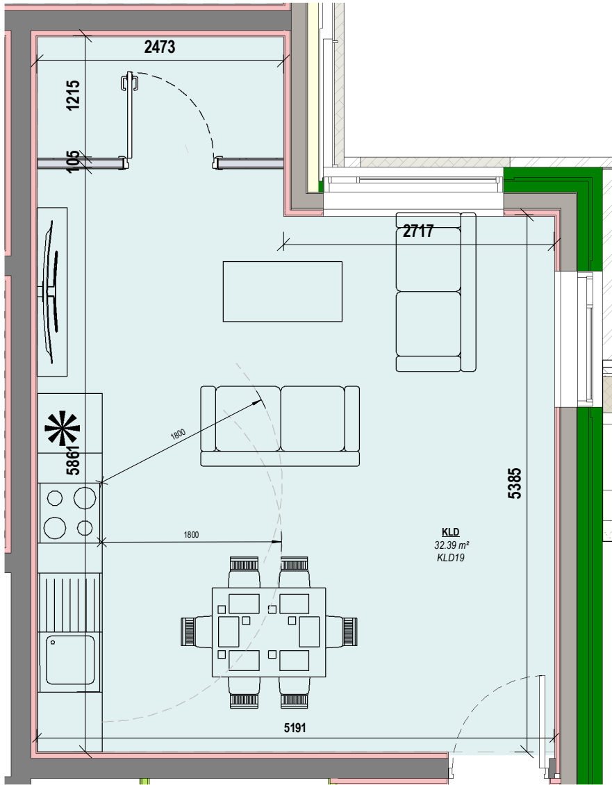
3 KLD19 Scale: 1 : 50
