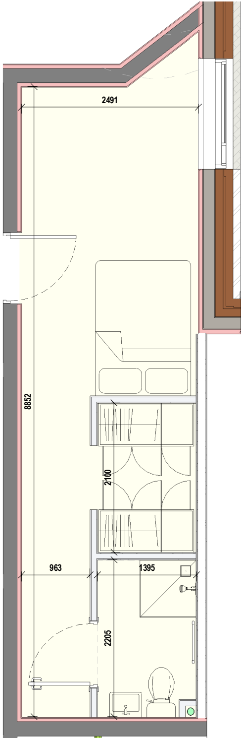
2 1B06 Scale: 1 : 50
