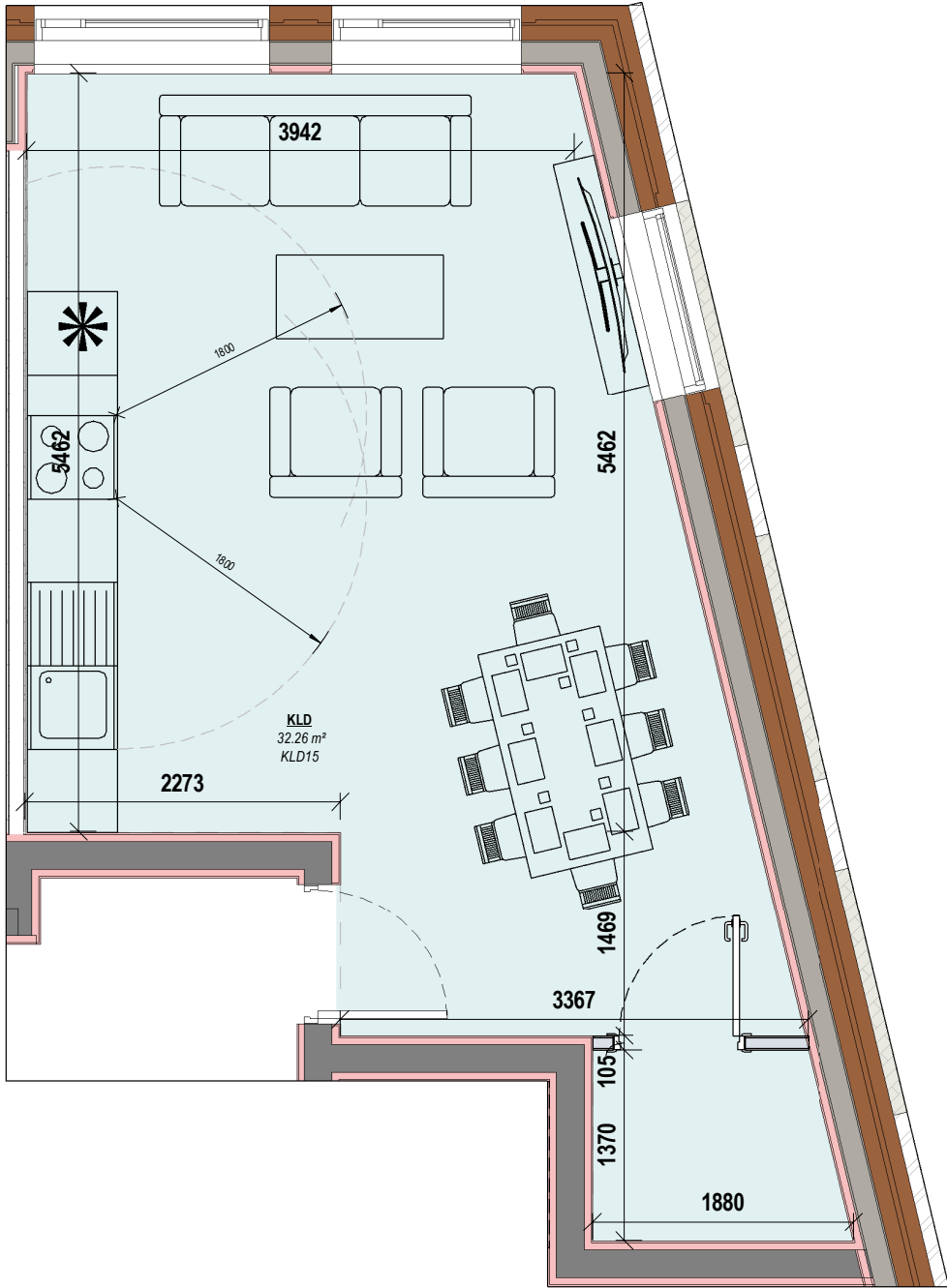
1 KLD15 Scale: 1 : 50
