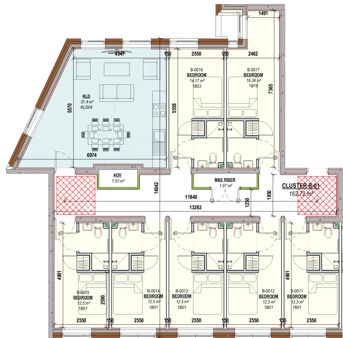
2 CLUSTER B-01 Scale: 1 : 100
