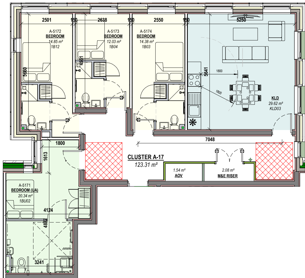
1 CLUSTER A-17 Scale: 1 : 100
