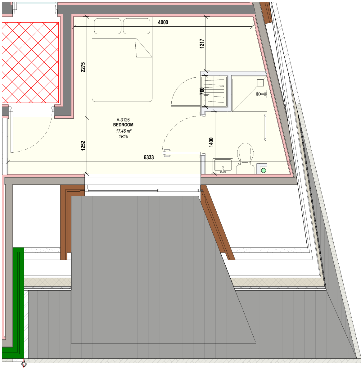
2 1B15 Scale: 1 : 50
