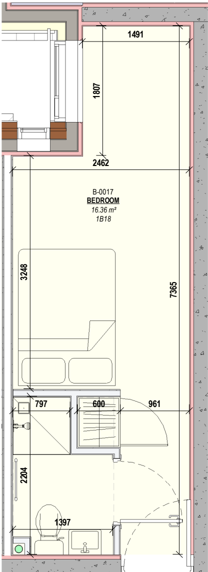
3 1B18 Scale: 1 : 50
