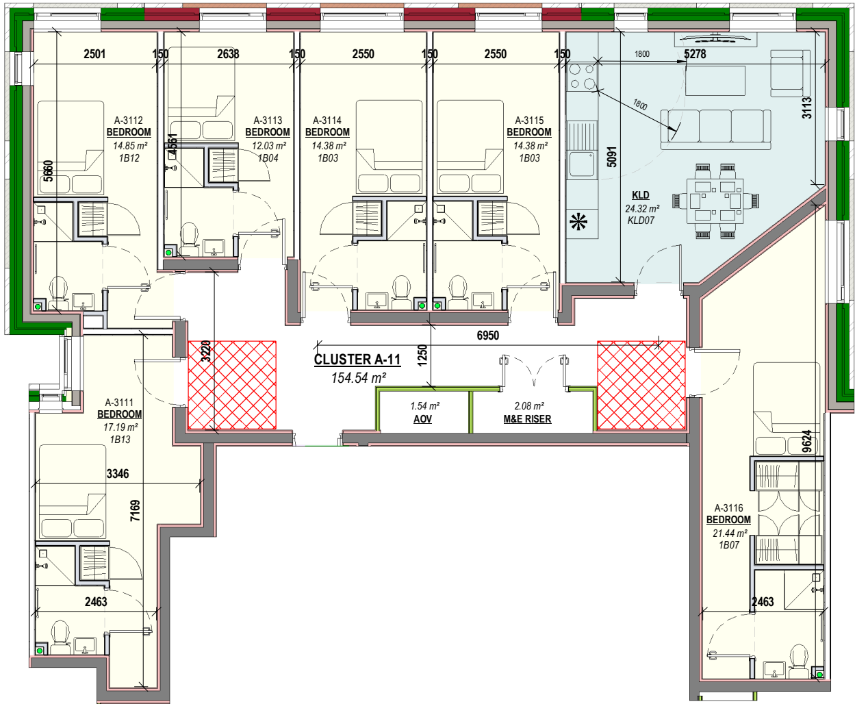
1 CLUSTER A-11 Scale: 1 : 100
