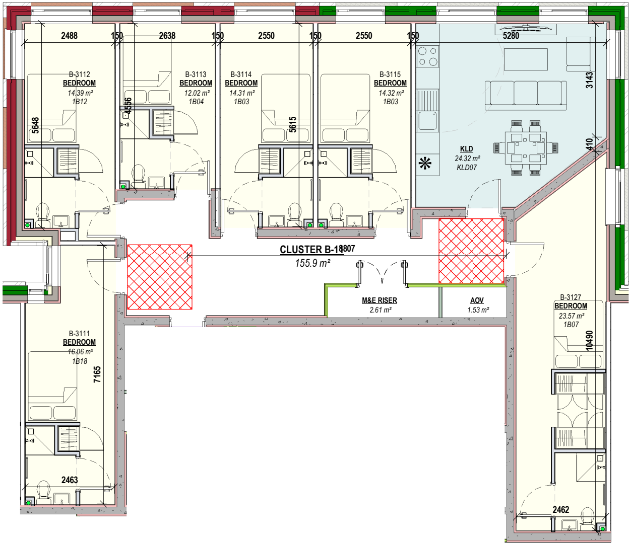
2 CLUSTER B-11 Scale: 1 : 100
