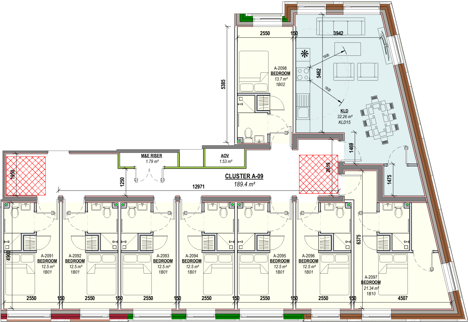
1 CLUSTER A-09 Scale: 1 : 100
