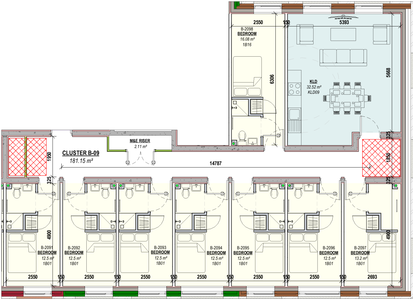
2 CLUSTER B-09 Scale: 1 : 100
