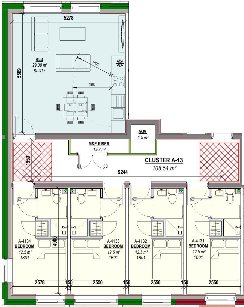
1 CLUSTER A-13 Scale: 1 : 100
