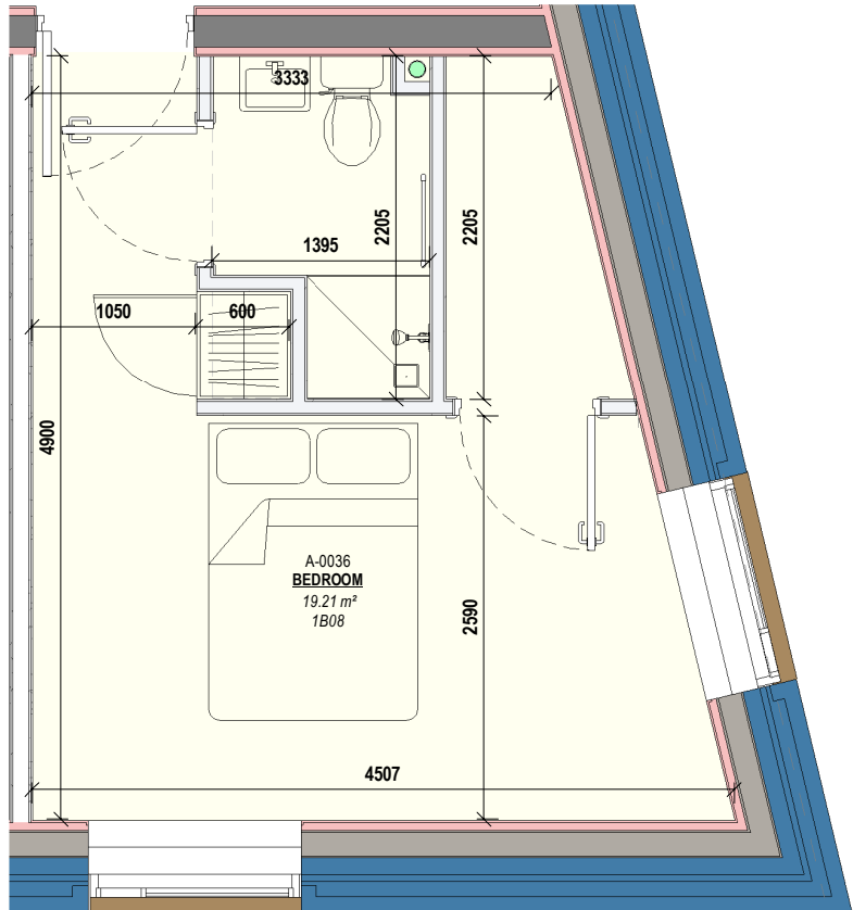
4 1B08 Scale: 1 : 50
