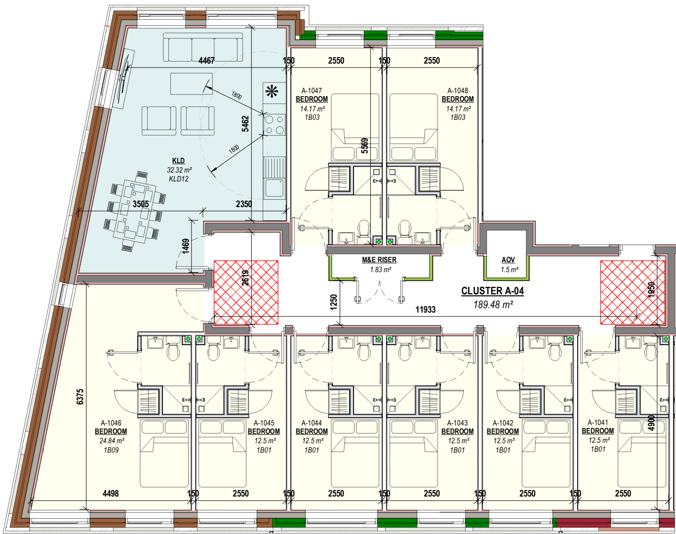
1 CLUSTER A-04 Scale: 1 : 100
