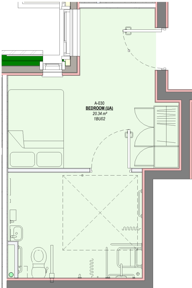
2 1BU02 Scale: 1 : 50
