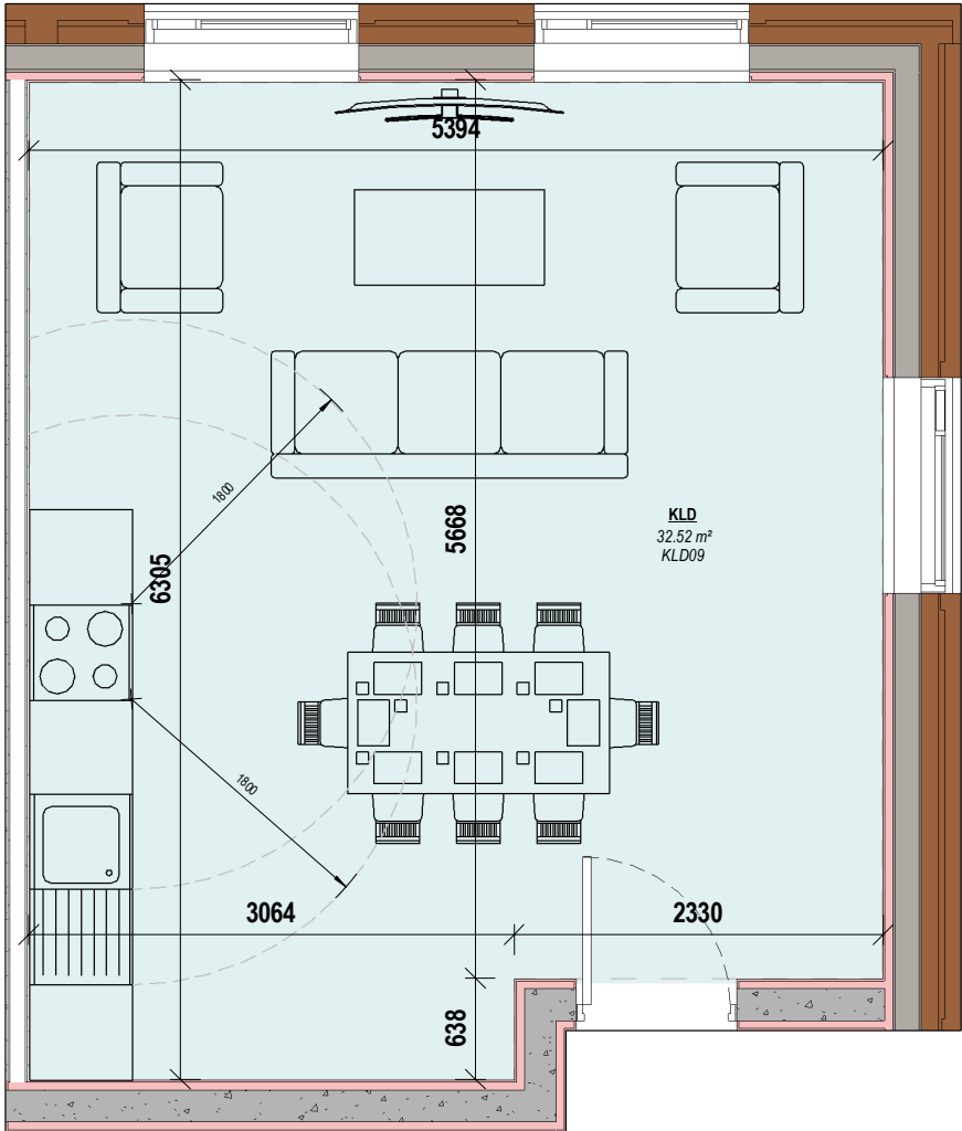
1 KLD09 Scale: 1 : 50
