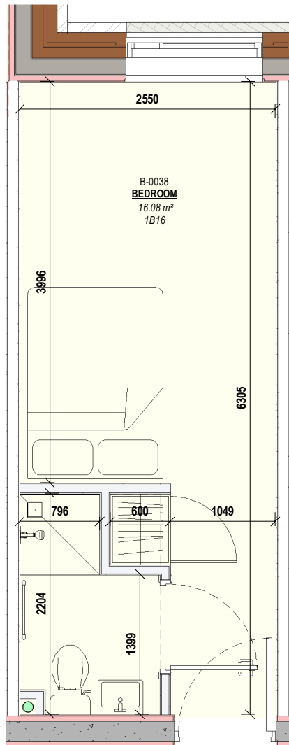
1 1B16 Scale: 1 : 50
