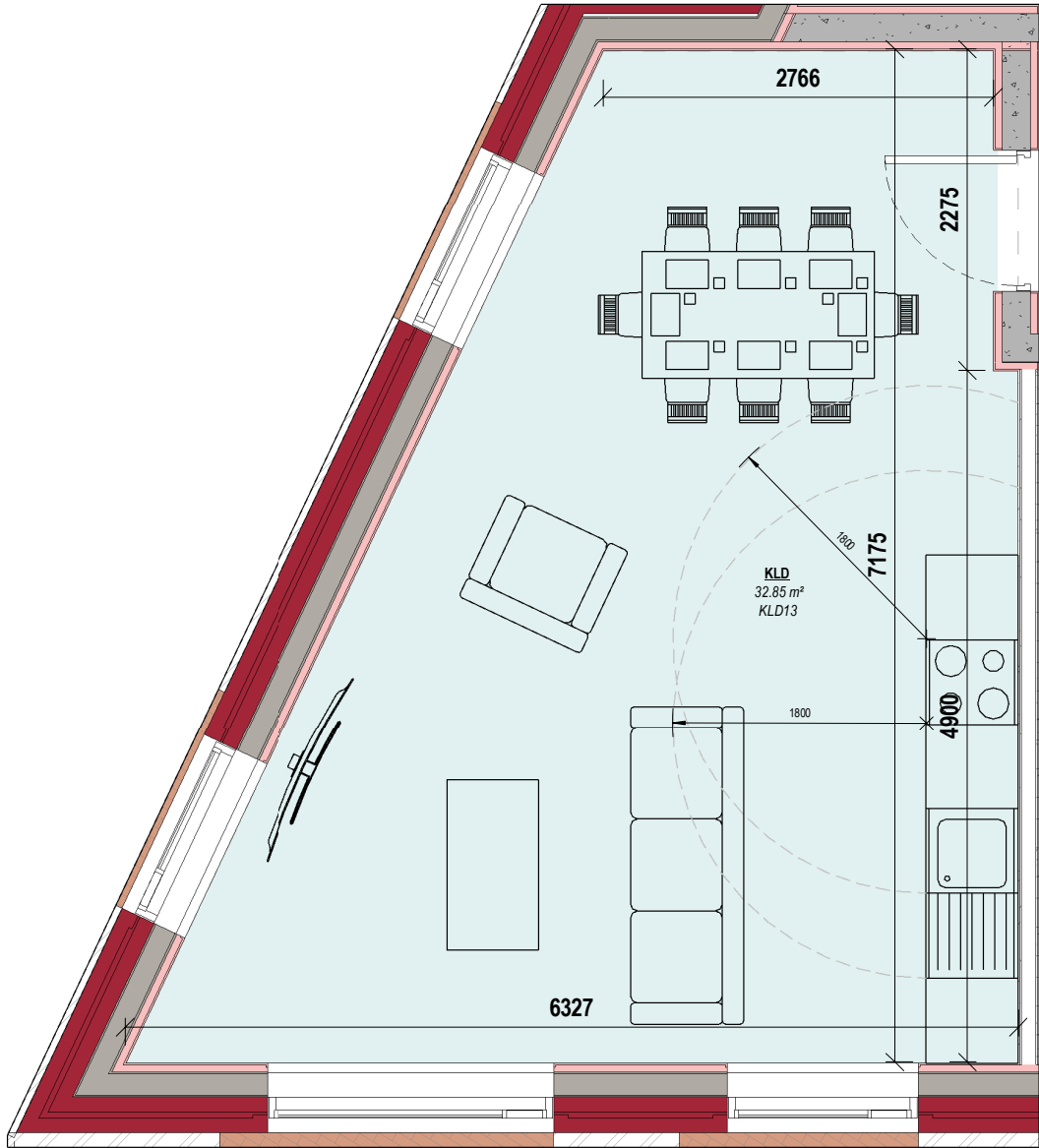
1 KLD13 Scale: 1 : 50
