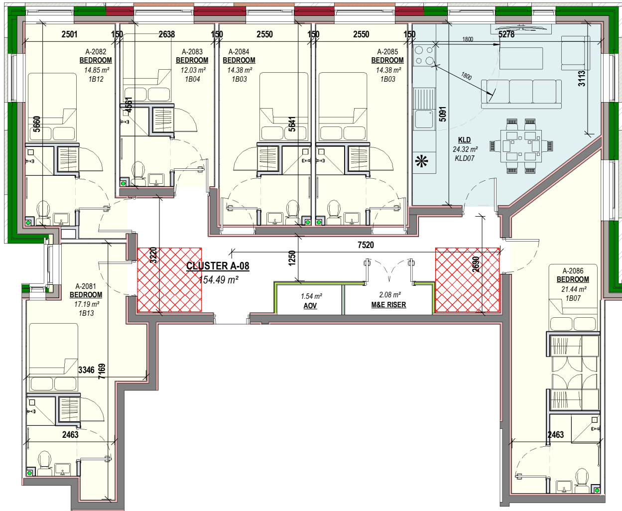
1 CLUSTER A-08 Scale: 1 : 100
