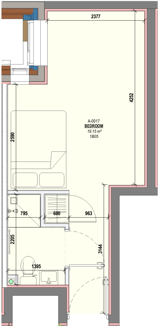
1 1B05 Scale: 1 : 50
