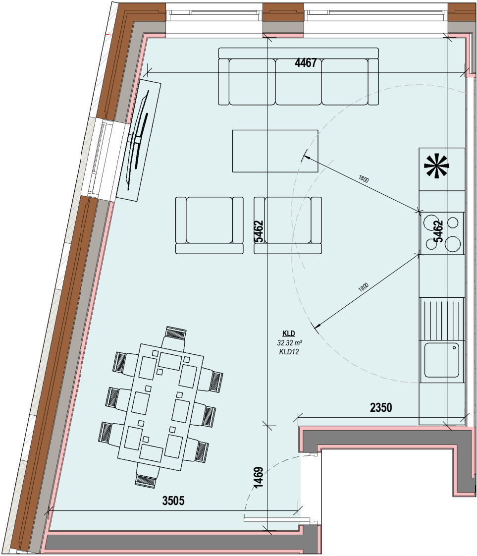
2 KLD12 Scale: 1 : 50
