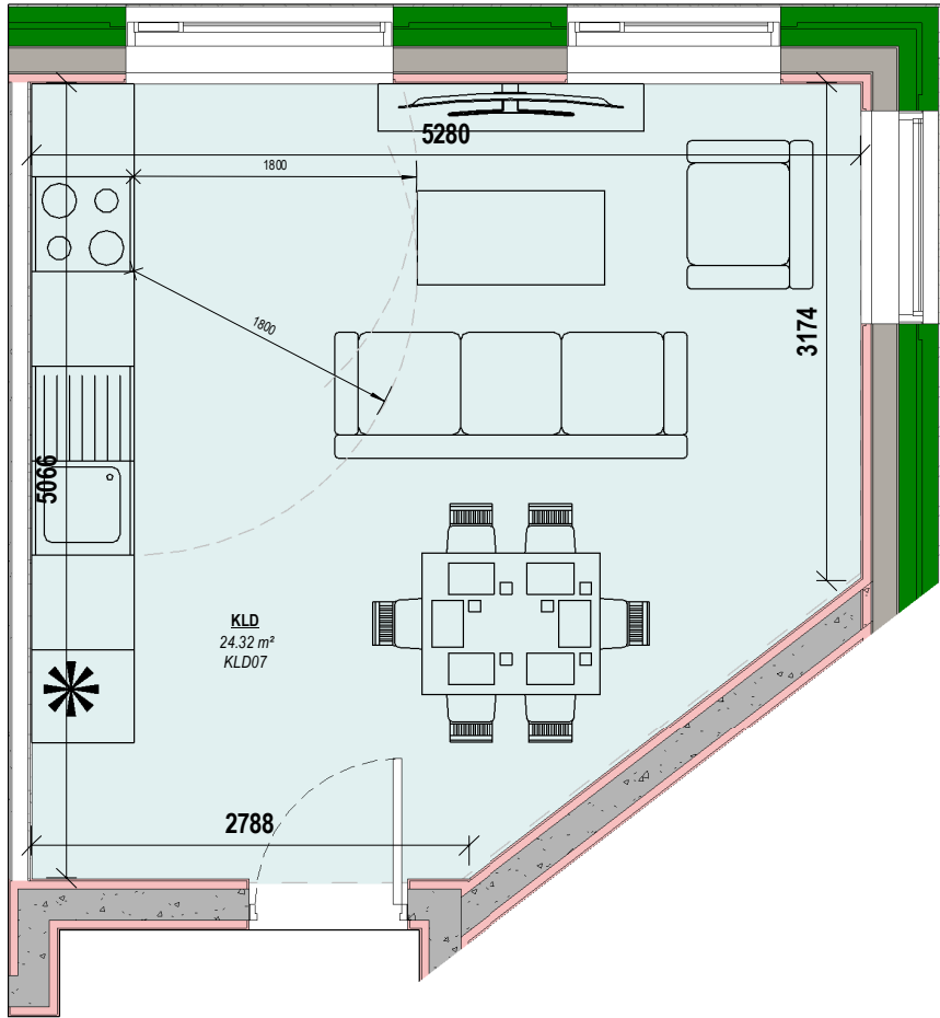
1 KLD07 Scale: 1 : 50
