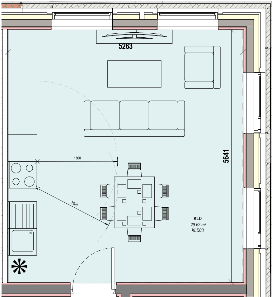
3 KLD03 Scale: 1 : 50
