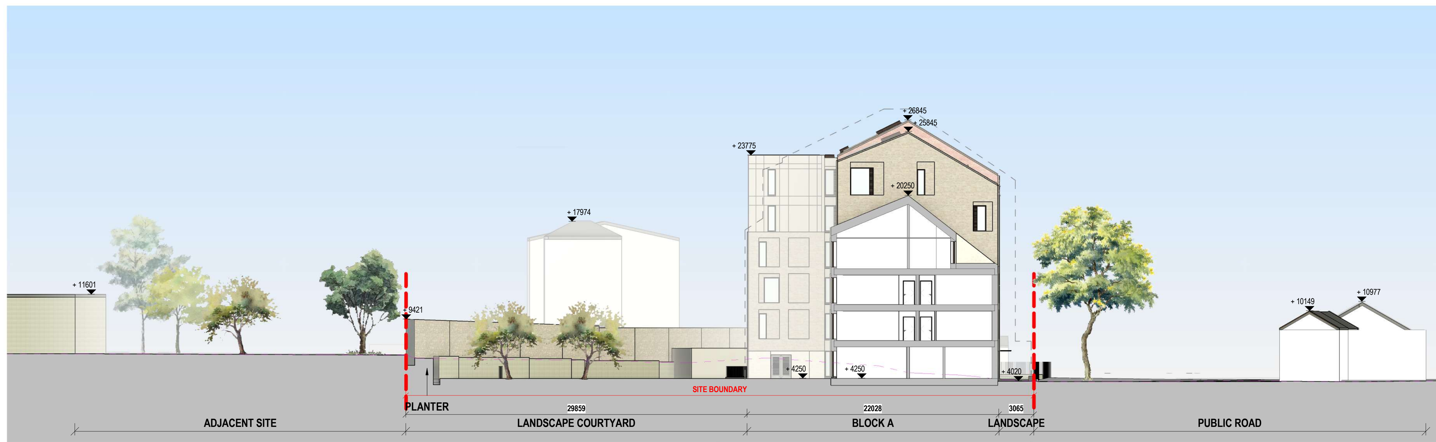
2 SITE - SECTION DD Scale: 1 : 200
