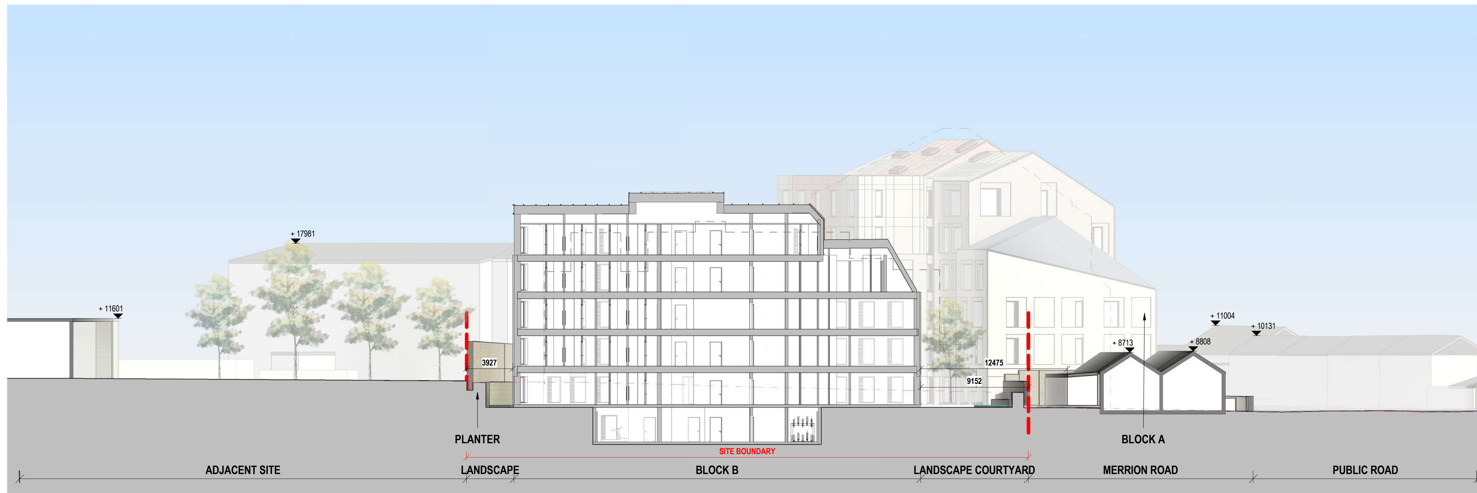
1 SITE - SECTION CC Scale: 1 : 200
